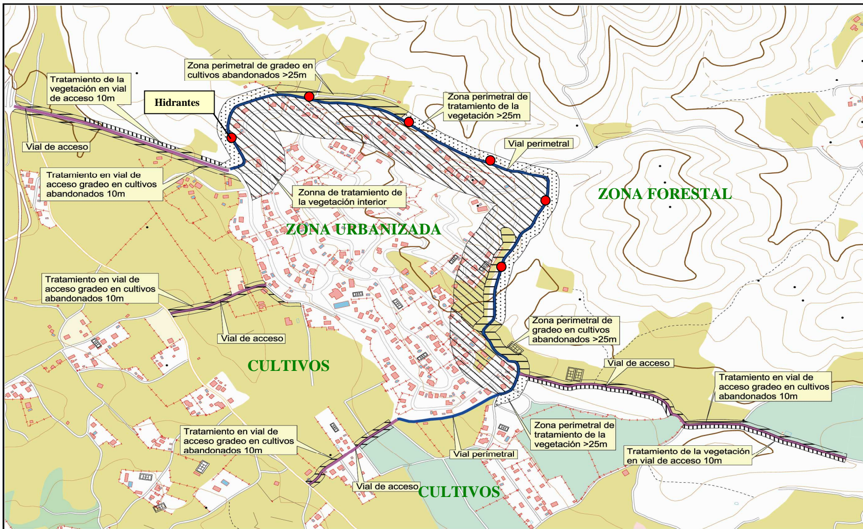
Figura 9. ESQUEMA GENERAL DE LAS ACTUACIONES A REALIZAR EN ZONAS URBANIZADAS.
