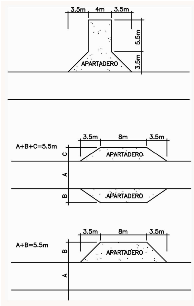
Figura 3. Función de cambio de sentido y apartadero
