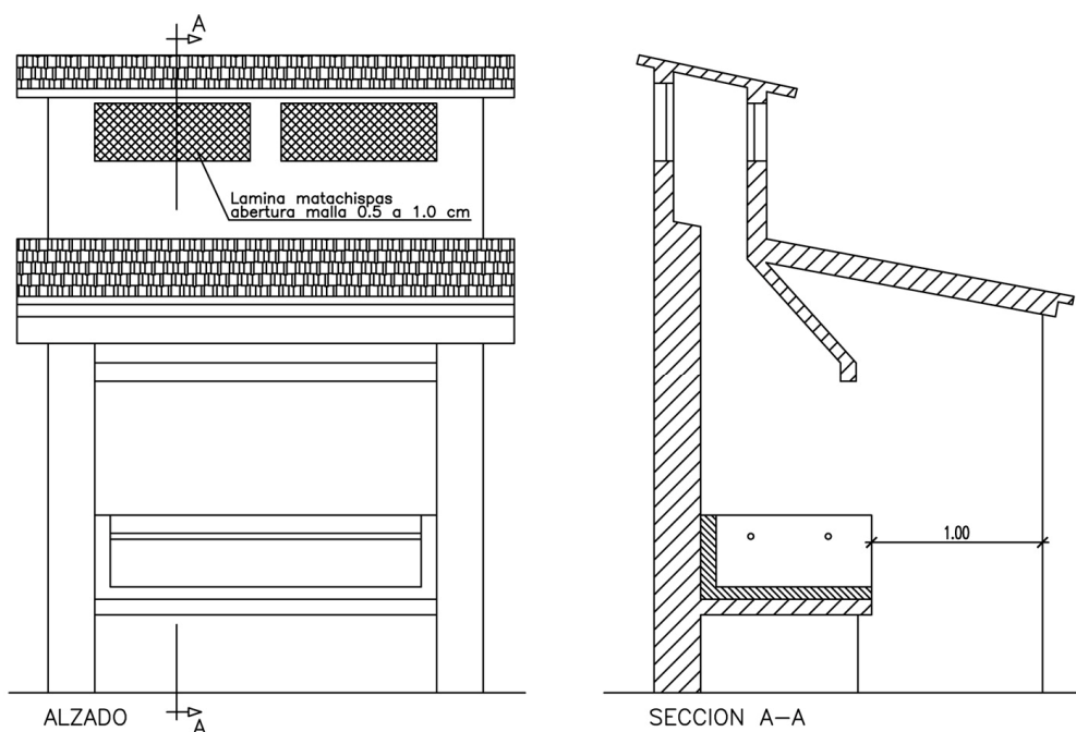
Figura 10. Alzados frontal y transversal de un paellero autorizable.
