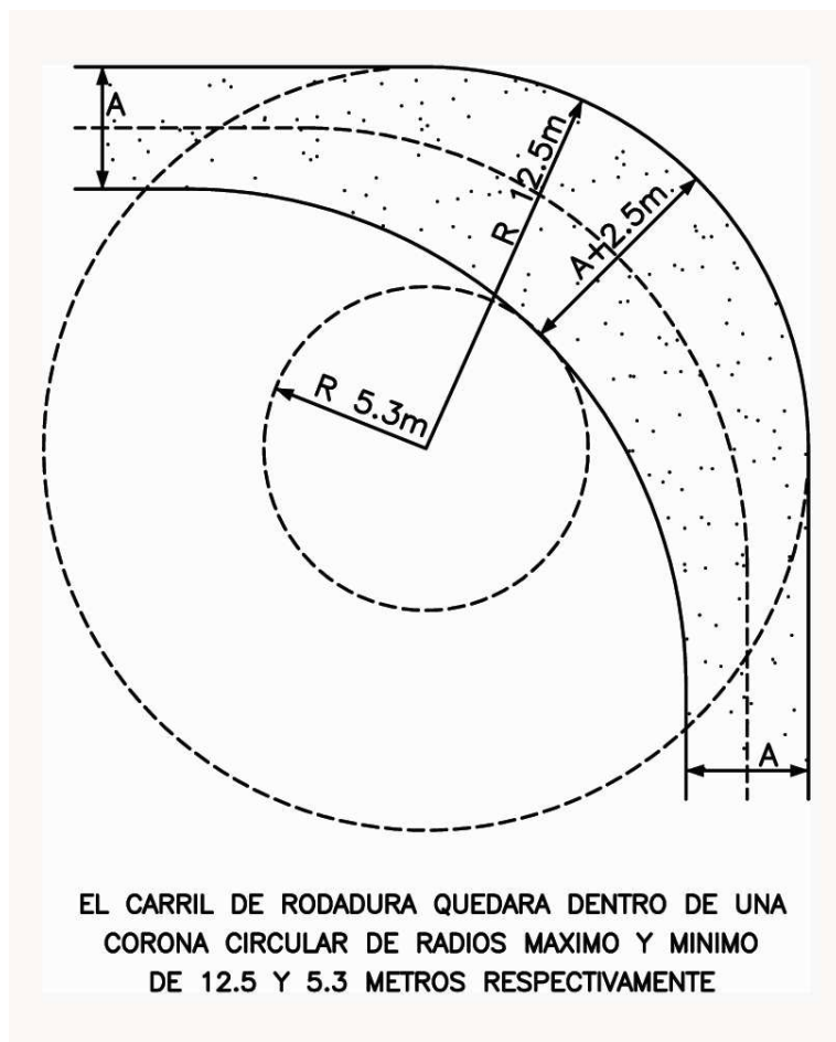
Figura 2. Sobrecanchos de la curva de radio mínimo.
