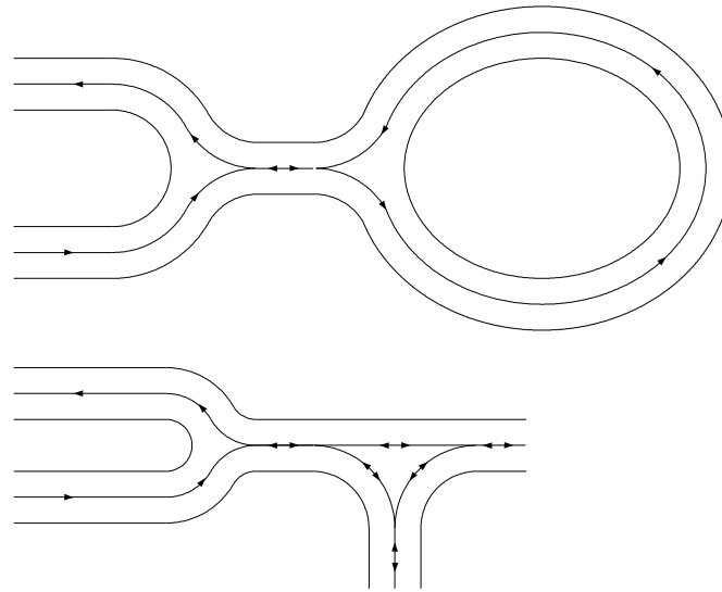
Figura 6. Soluciones para permitir el cambio de sentido a los vehículos en lugares comprometidos para su paso.
