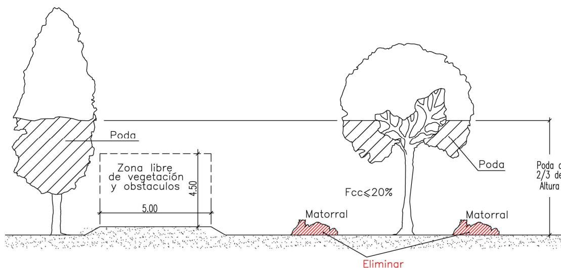
Figura 7. Alzado del tratamiento de la vegetación en los viales de acceso.
