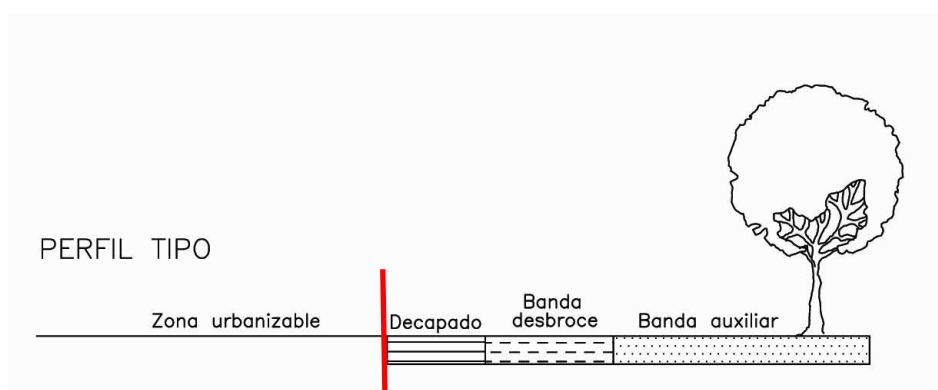
Figura 1. Alzado de Área Cortafuegos perimetral a urbanización.
